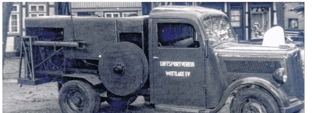
Präsentation des ersten Seilwindfahrzeuges im Jahre 1961.
